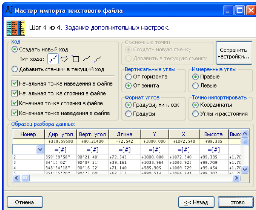
Четвертый шаг мастера импорта текстового файла
