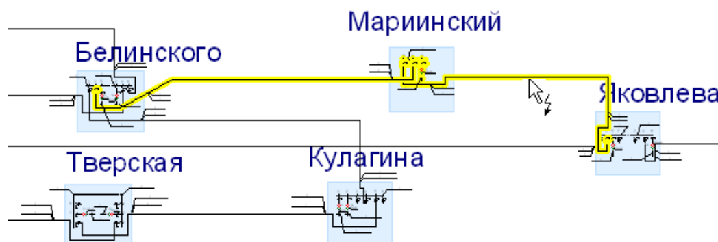
Указание расчётной схемы
