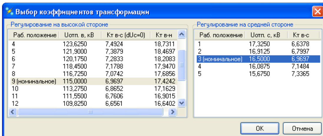
Выбор коэффициентов трансформации для трёхобмоточного трансформатора
