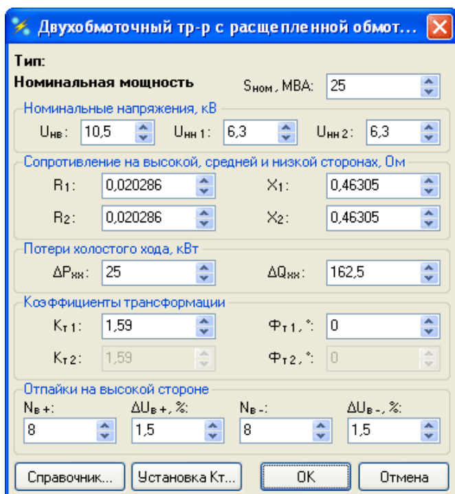
Параметры двухобмоточного трансформатора с расщеплённой обмоткой
